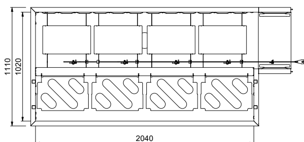
Dessus
